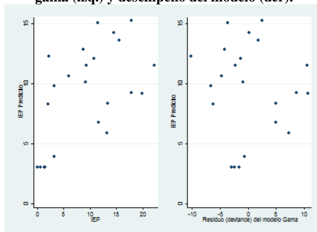
Figura 2: Valores predichos por el modelo gama (izq.) y desempeño del modelo (der).
