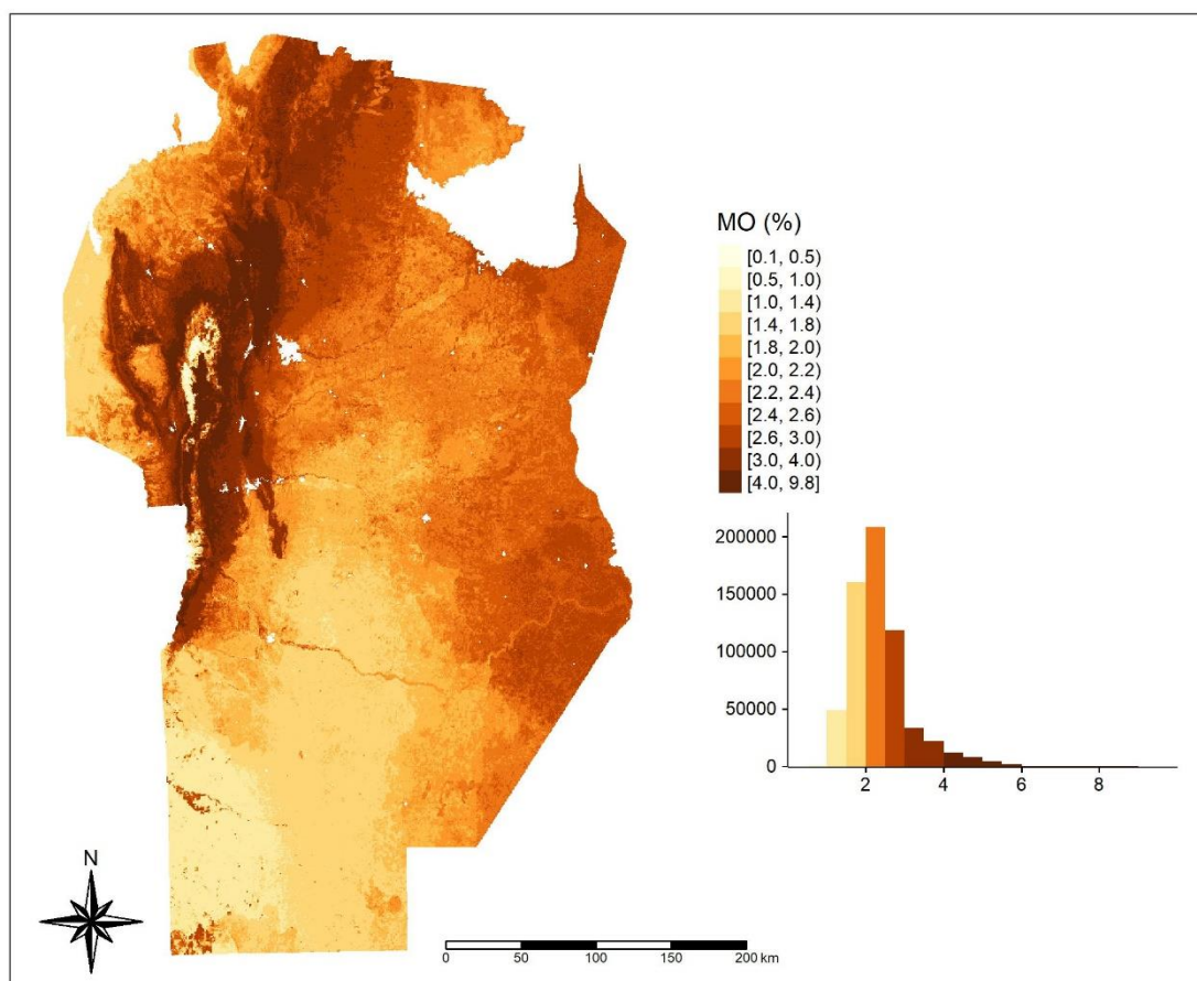
Figura 2. Mapa de predicción de la materia orgánica (MO) del suelo en la provincia de Córdoba, 2020.
