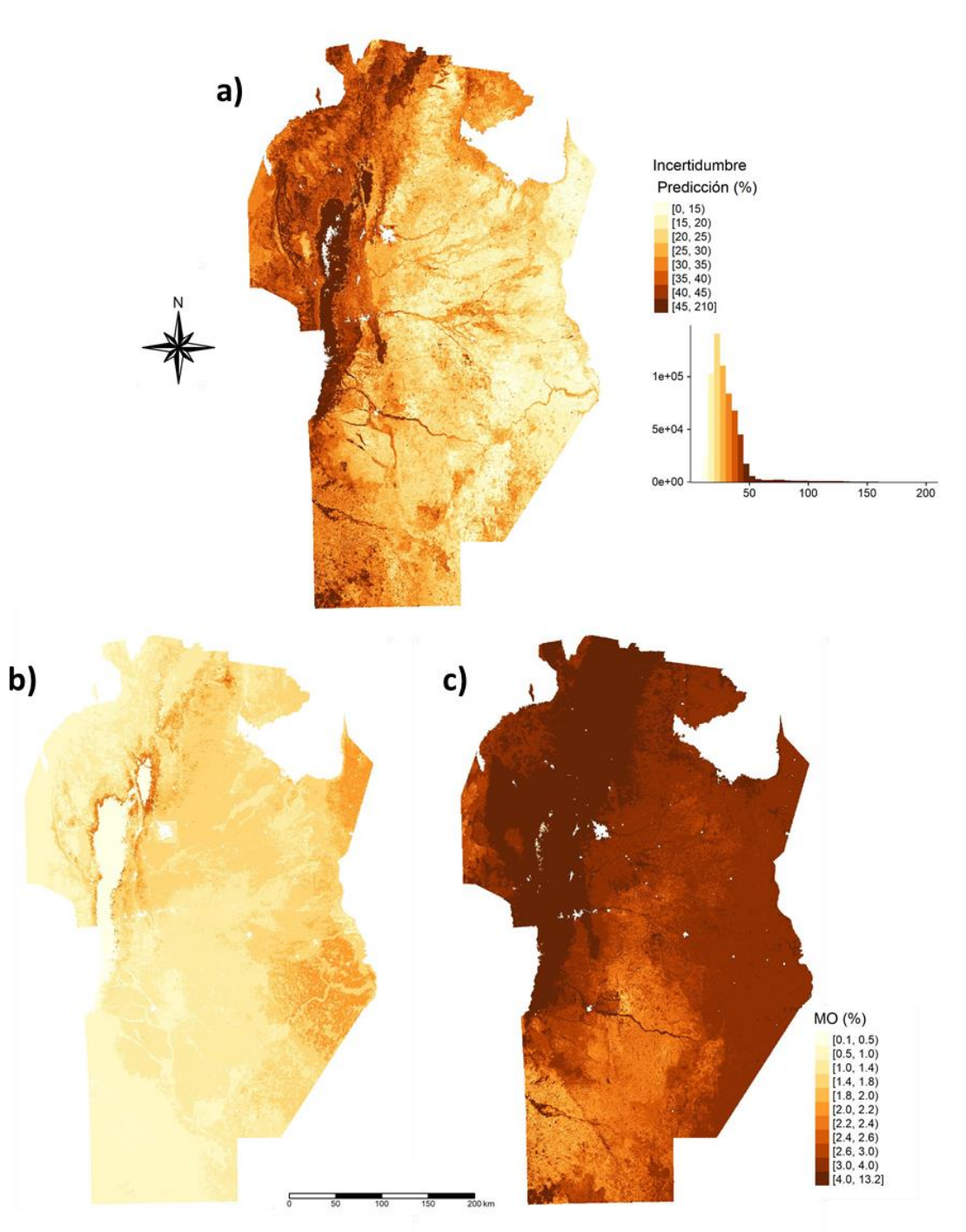
Figura 3. Mapa de incertidumbre de predicción de la materia orgánica (MO) del suelo en la Provincia de Córdoba. a) Incertidumbre de predicción relativa al valor predicho, b) Límite Inferior de Predicción, Cuantil 0,05, c) Límite Superior de Predicción, Cuantil 0,95.
